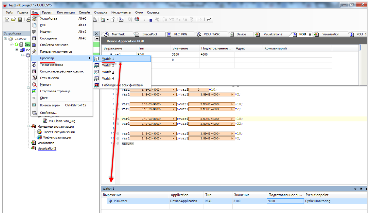
Рисунок 8.15 – Создание списка просмотра
