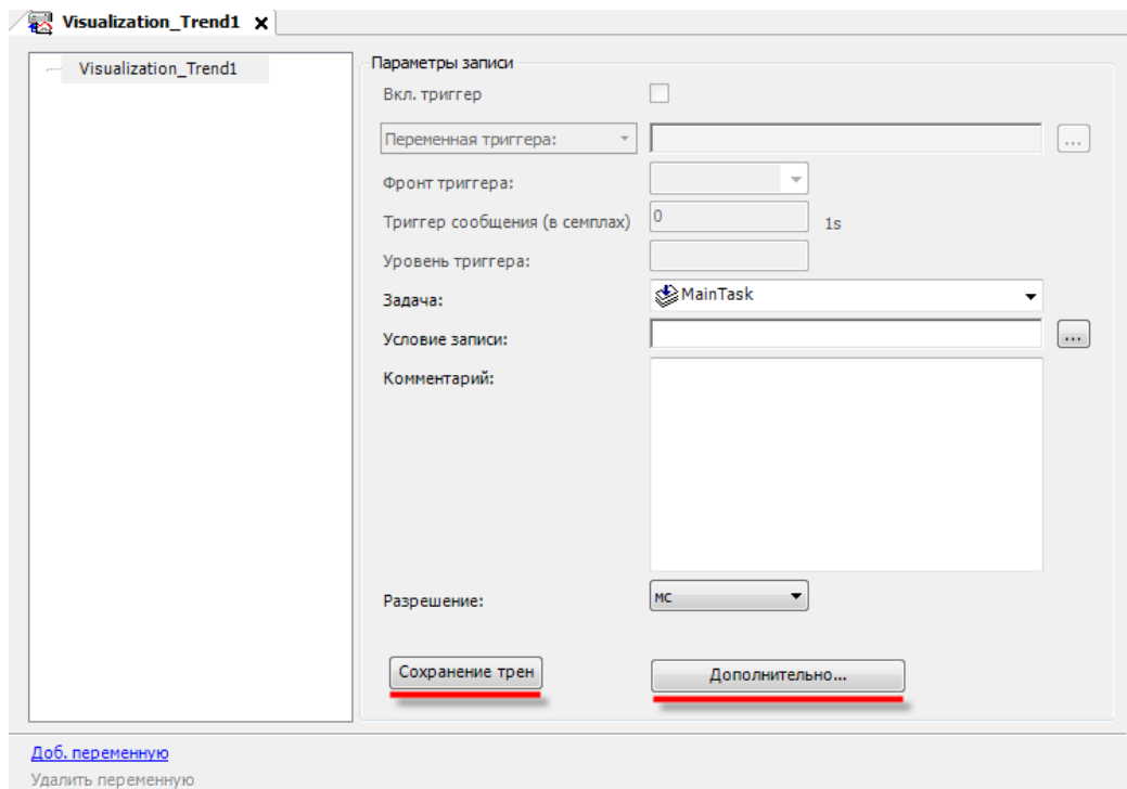
Рисунок 7.70 – Конфигурация тренда
