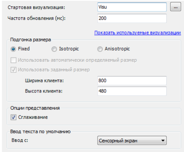
Рисунок 10.159 – Настройки таргет-визуализации
